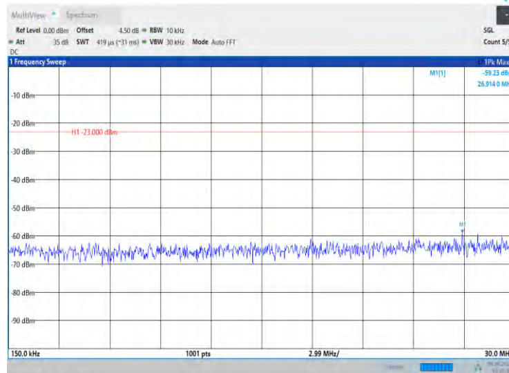
Band66-20MHz-QPSK-132072-1RB#0-Range2:0.15~30MHz
