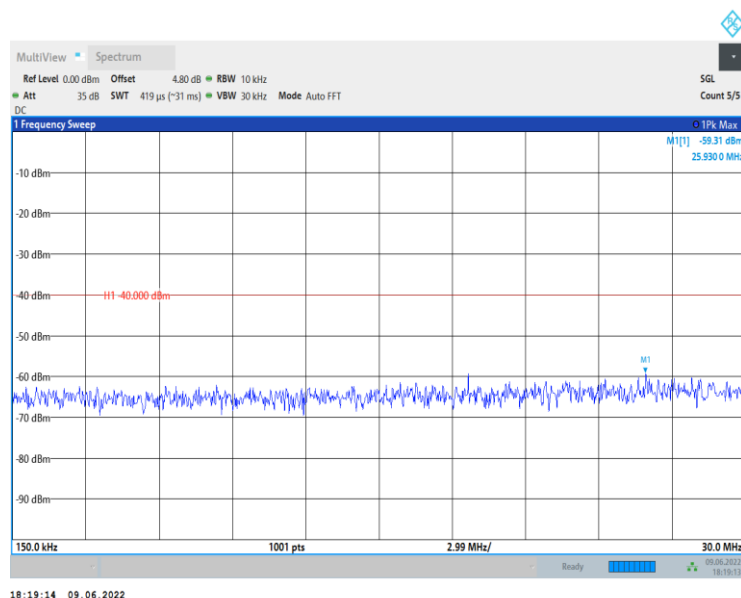
Band30-10MHz-QPSK-27710-1RB#0-Range2:0.15~30MHz
