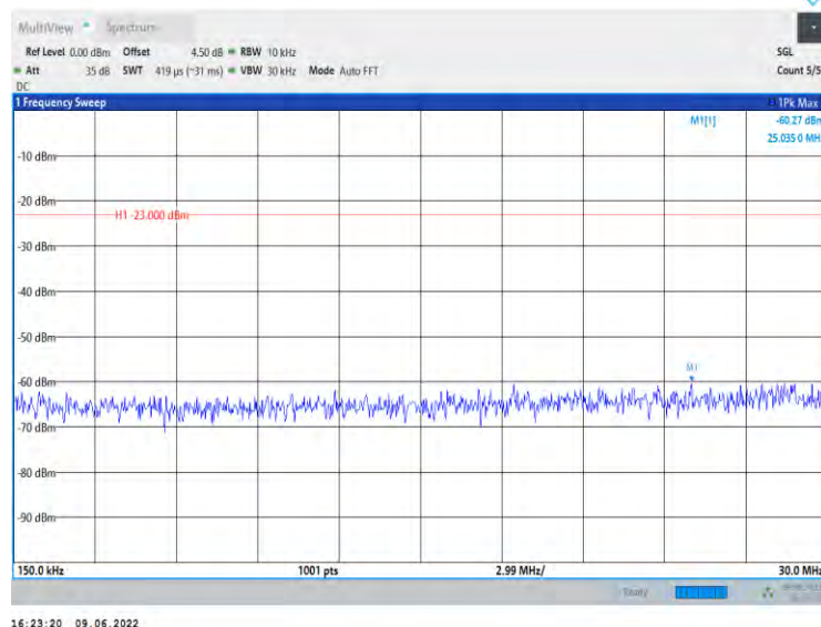
Band25-20MHz-QPSK-26140-1RB#0-Range2:0.15~30MHz
