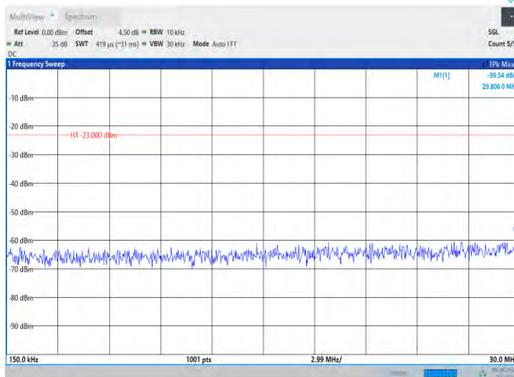
Band4-20MHz-QPSK-20050-1RB#0-Range2:0.15~30MHz
