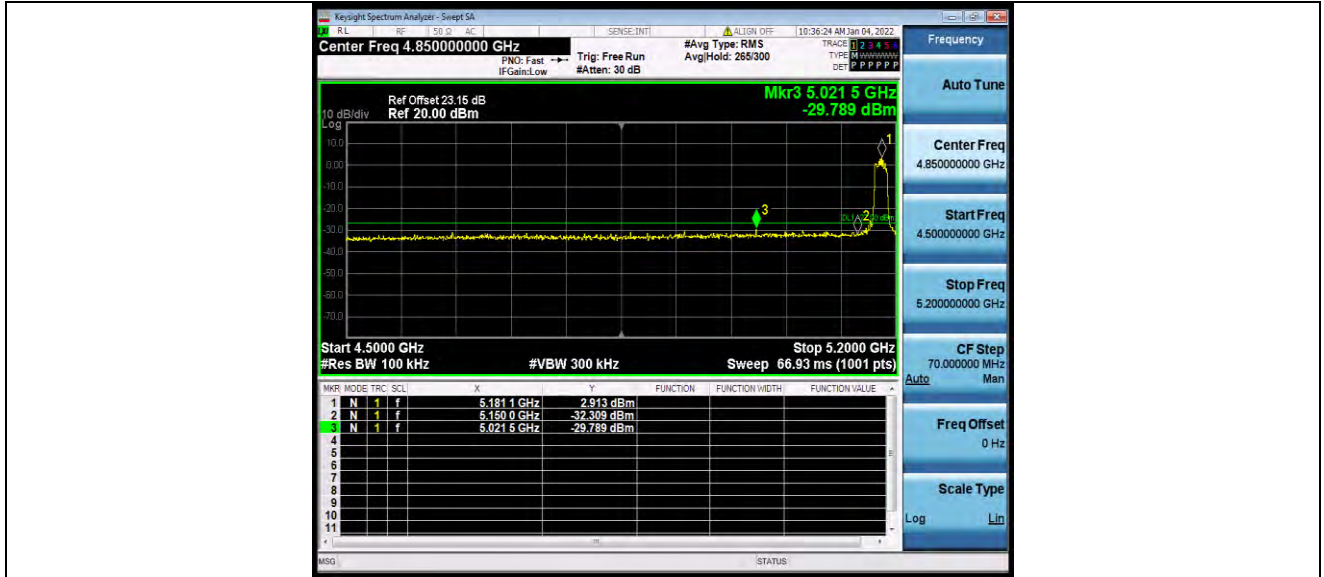
11A_Ant1_Low_5180
