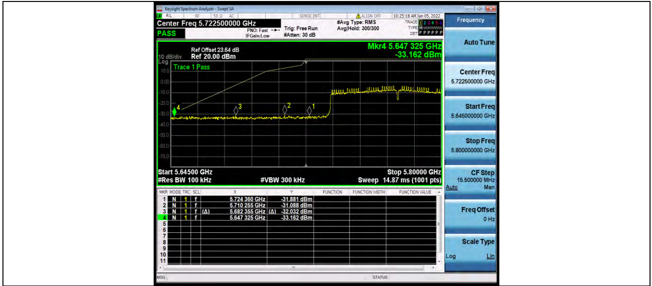
11AC80SISO_Ant1_Low_5775
