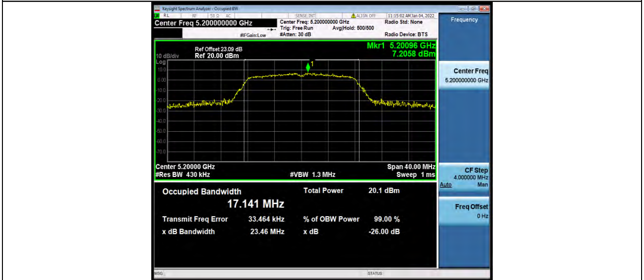
11A_Ant1_5200
