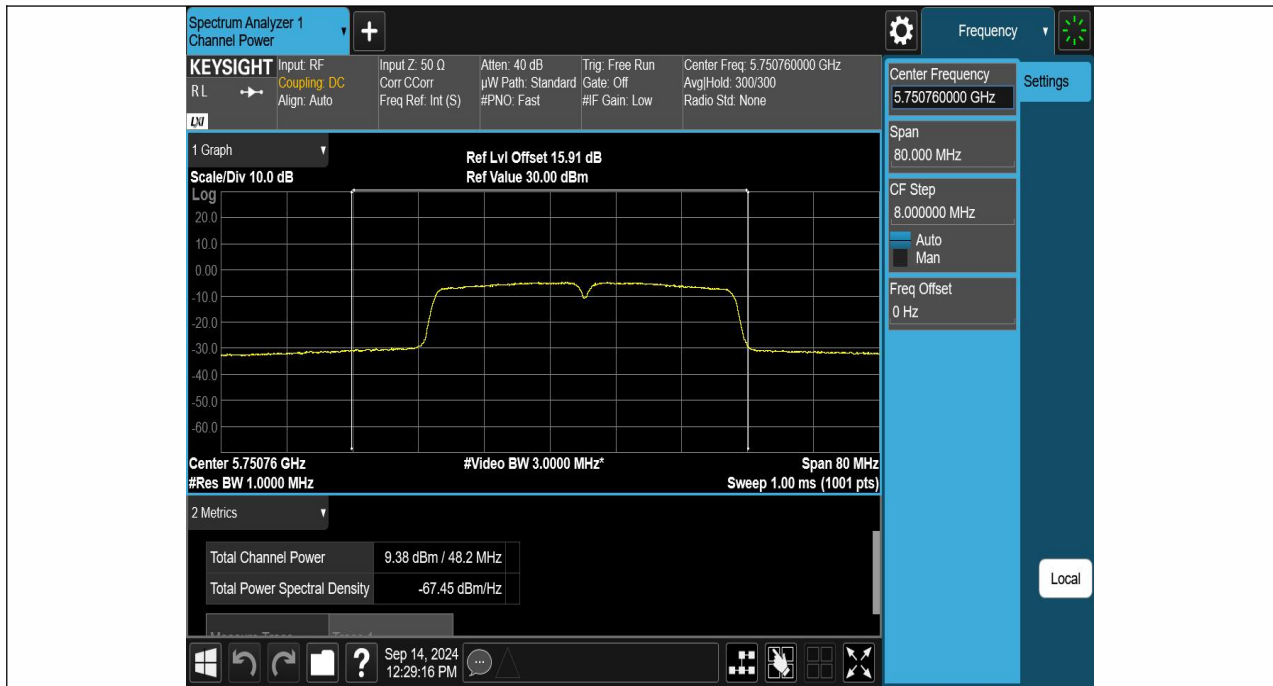
11N40SISO-Ant1-5755-PASS
