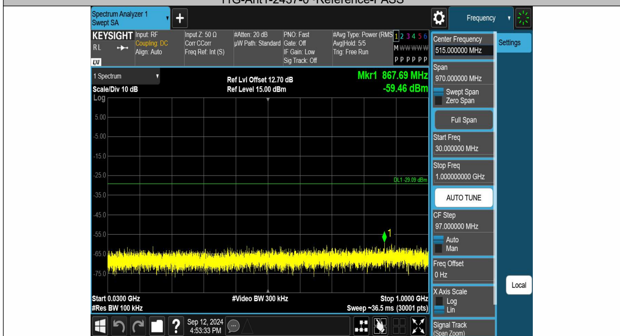
11G-Ant1-2437-30~1000-PASS
