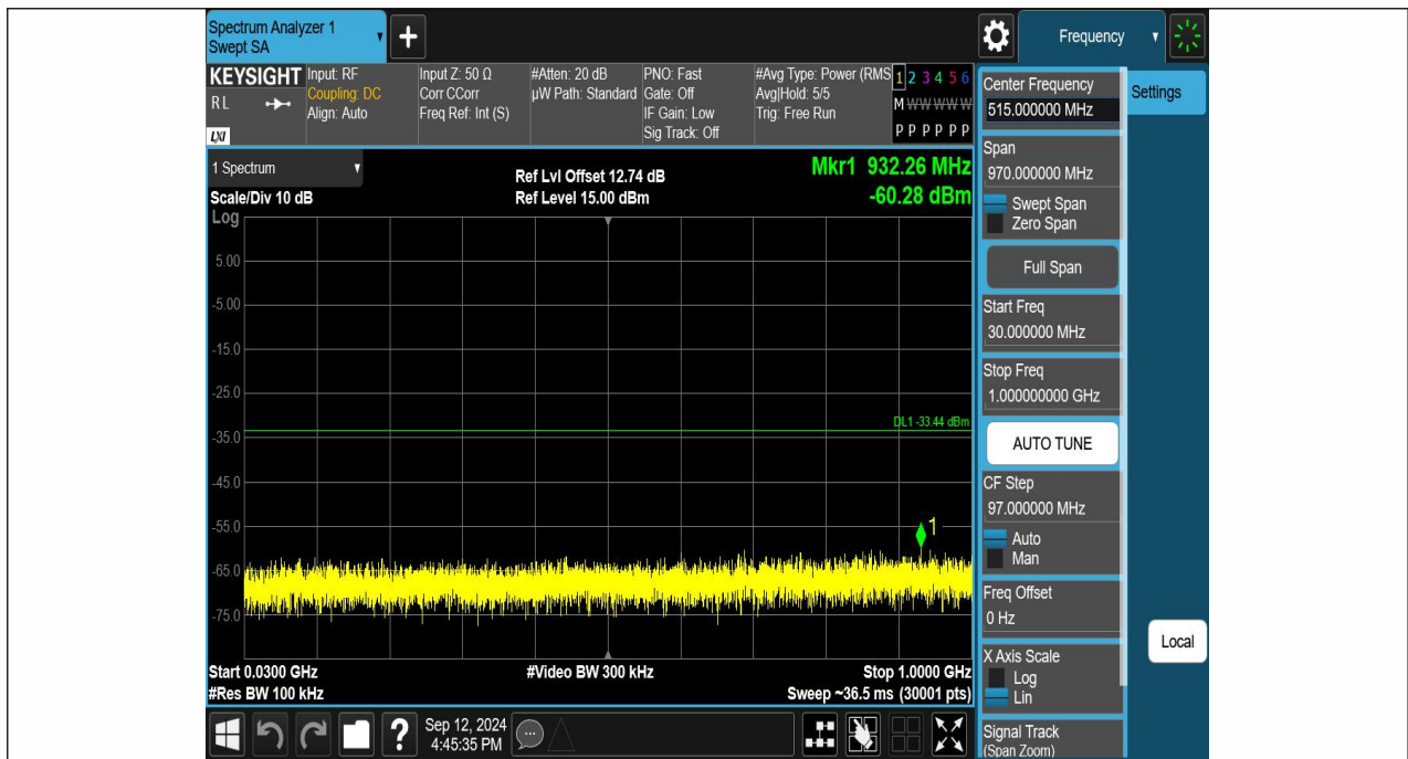
11G-Ant1-2412-30~1000-PASS
