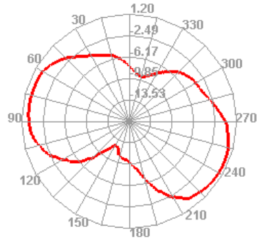
2450.000MHz E2
