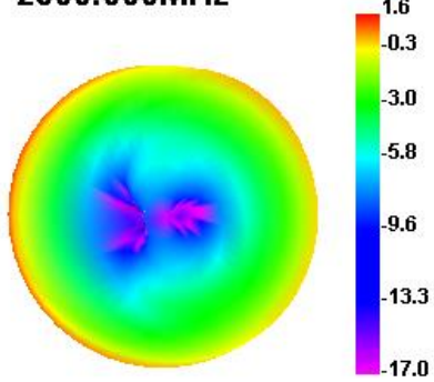
2500.000MHz
