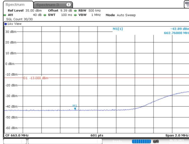
Band71-20MHz-QPSK-133222-1RB#99
