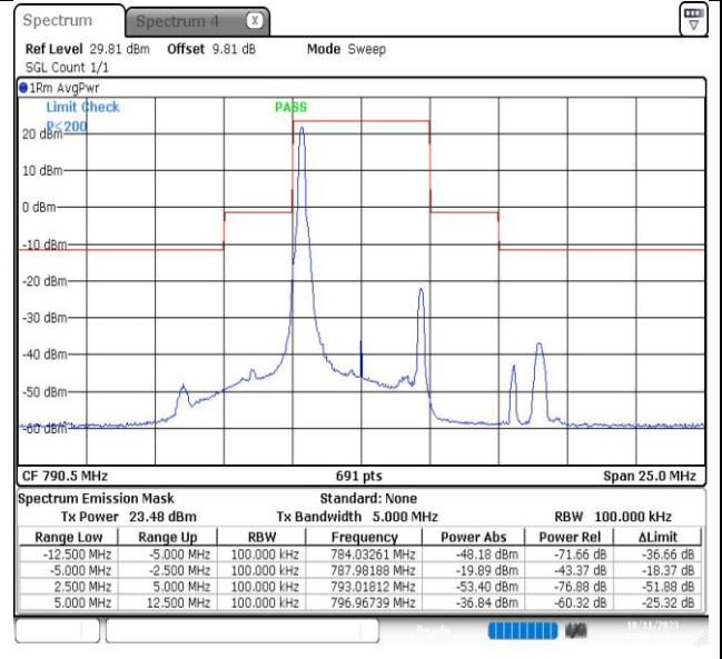
NTNV-Band14-5MHz-QPSK-23305-1RB#0--5.00--2.50-PASS
