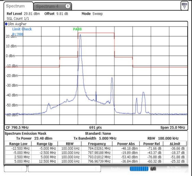
NTNV-Band14-5MHz-QPSK-23305-1RB#0--5.00--2.50-PASS
