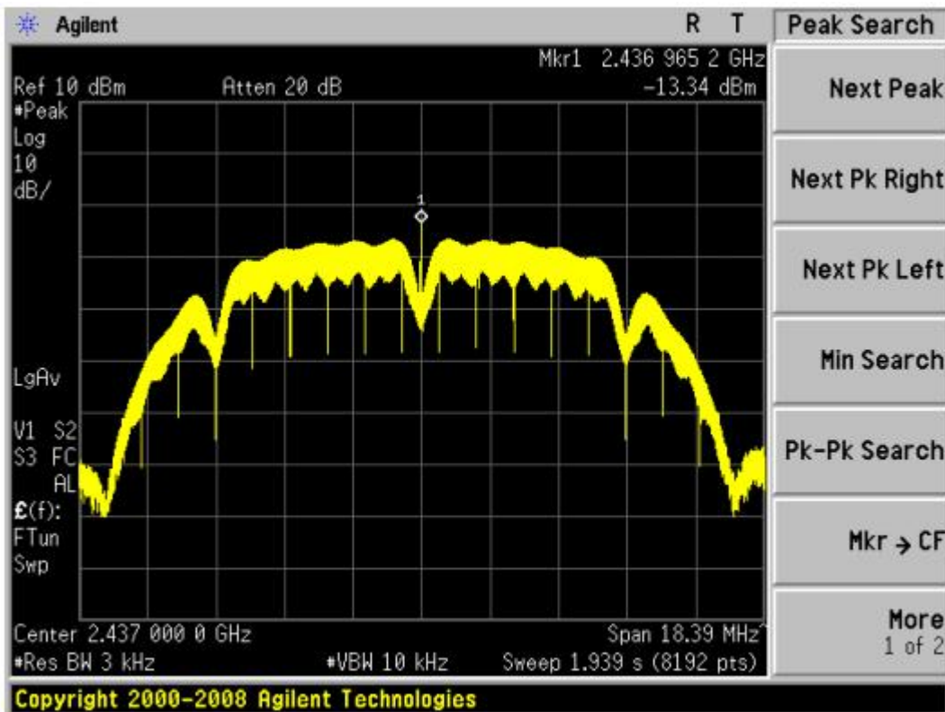
802.11b-2437MHz
