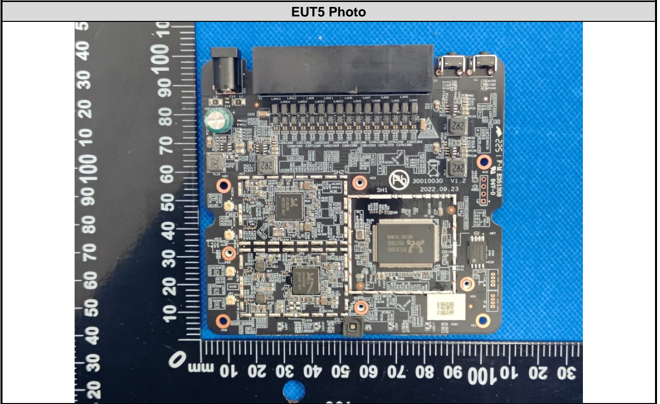
EUT5 Photo
