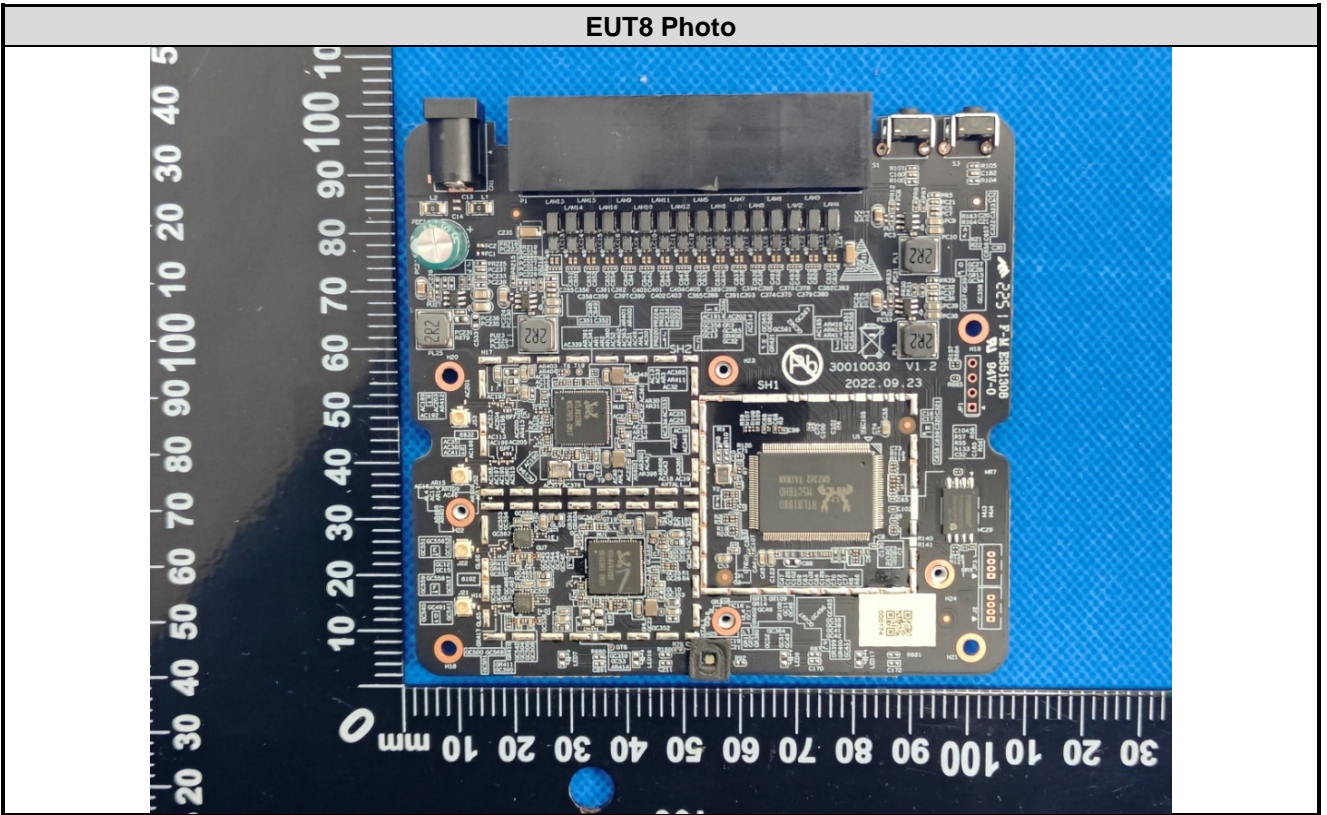
EUT8 Photo
