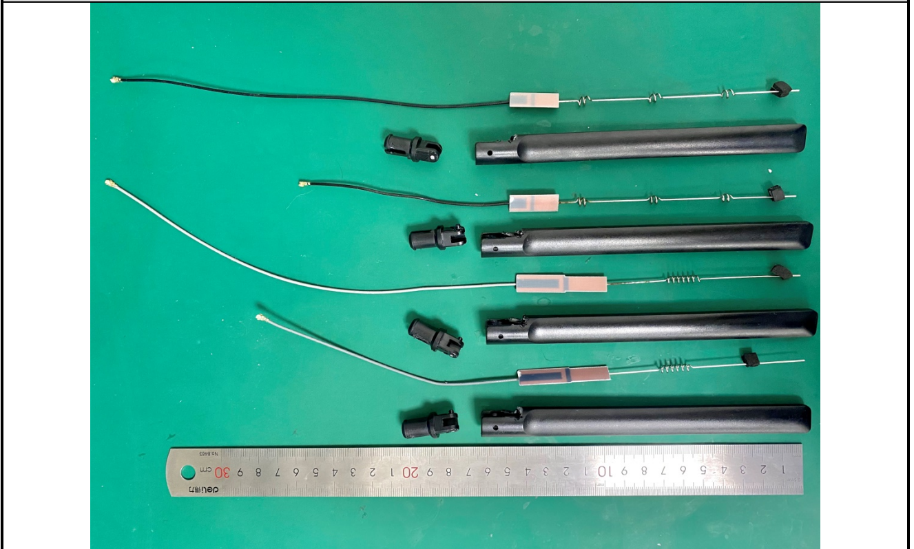
EUT5 Photo
