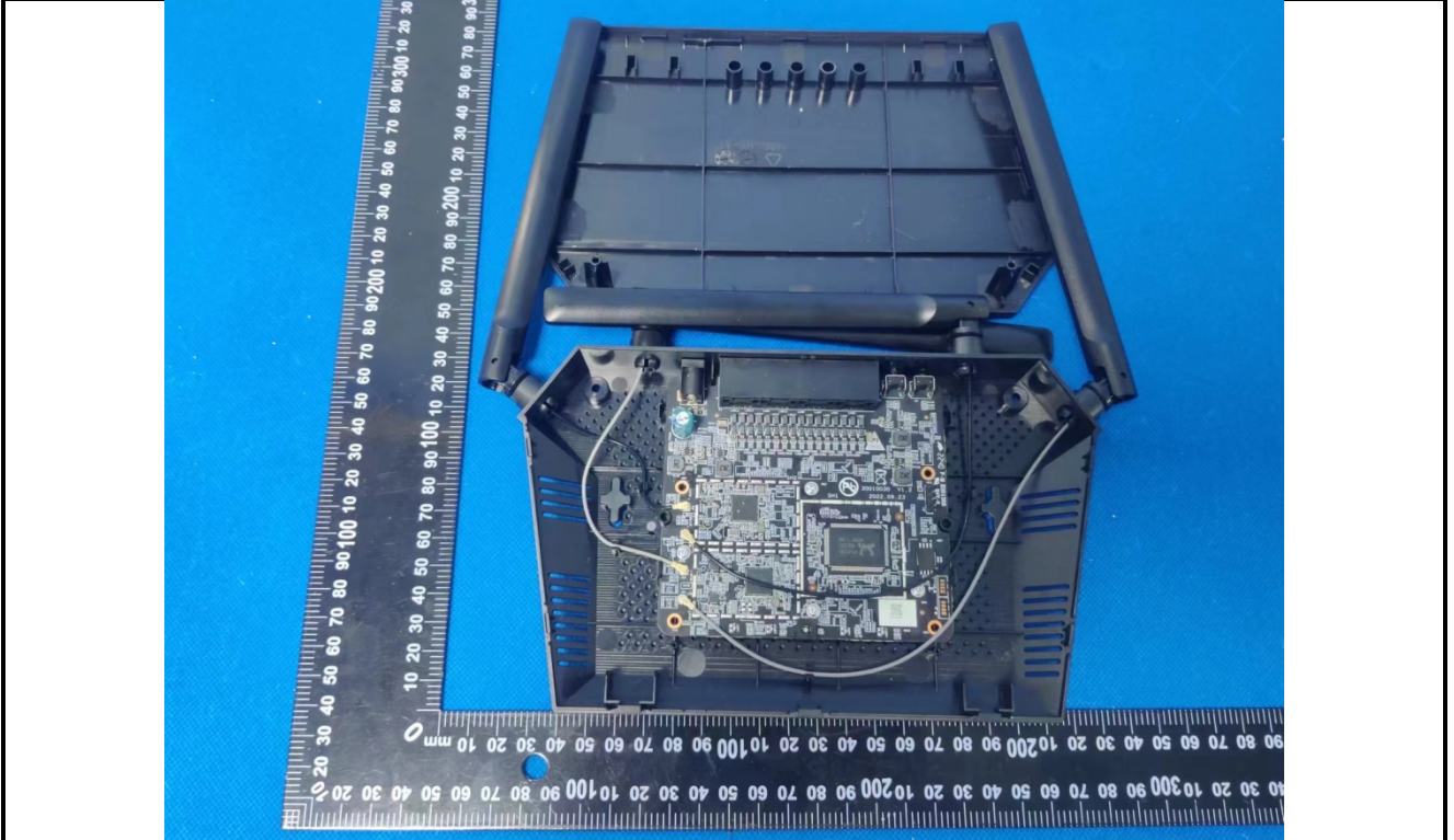
EUT5 Photo
