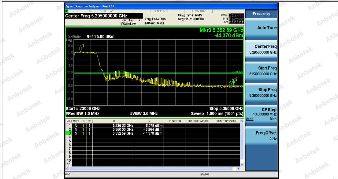
11N40SISO_Ant1_Low_5270
