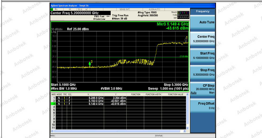
11AC80SISO_Ant1_Low_5290
