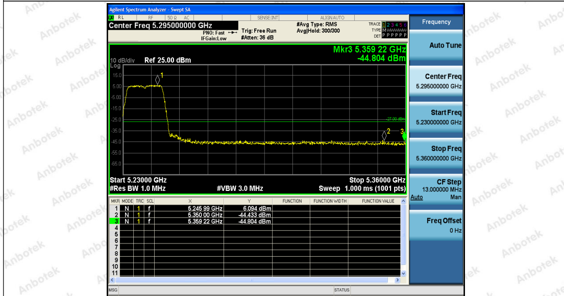
11A_Ant1_Low_5260
