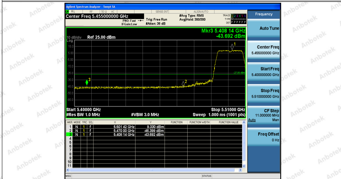
11A_Ant2_Low_5500
