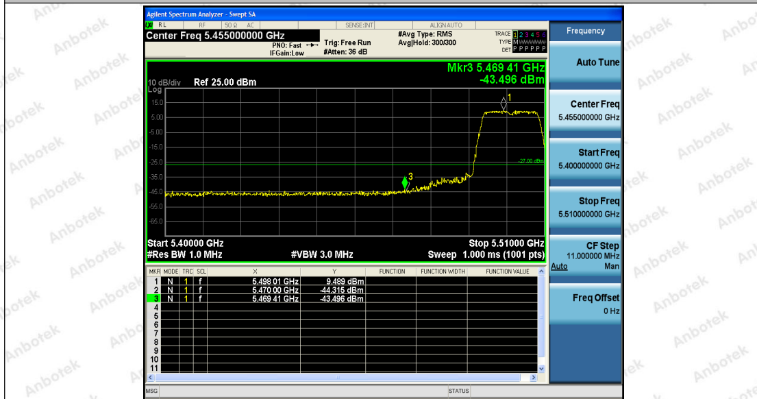
11A_Ant2_Low_5500
