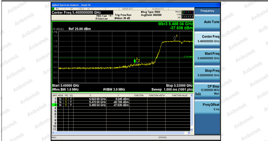
11N40SISO_Ant2_Low_5510
