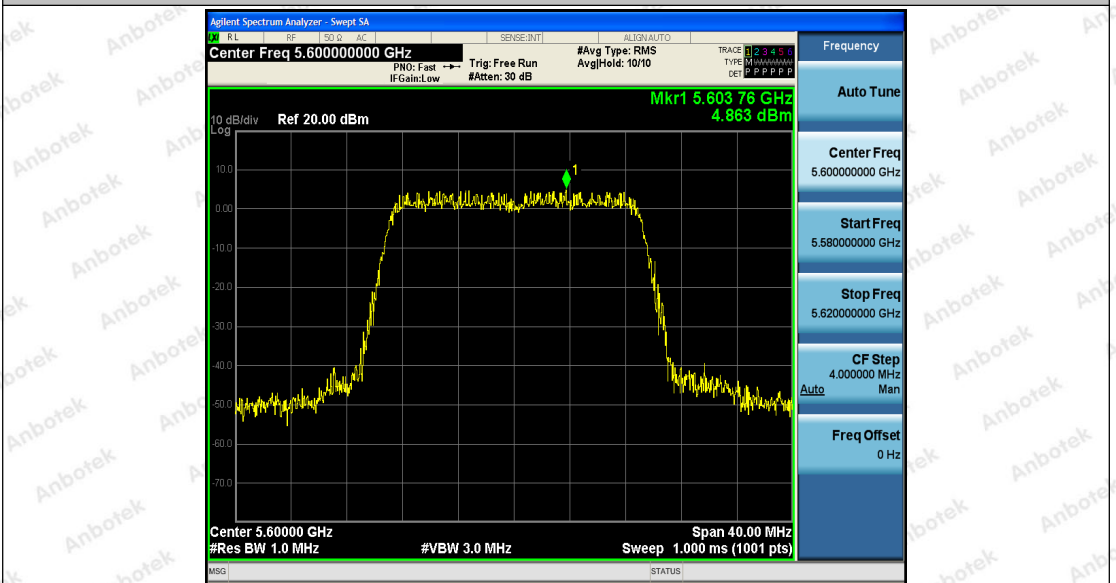
11N20SISO_Ant2_5600
