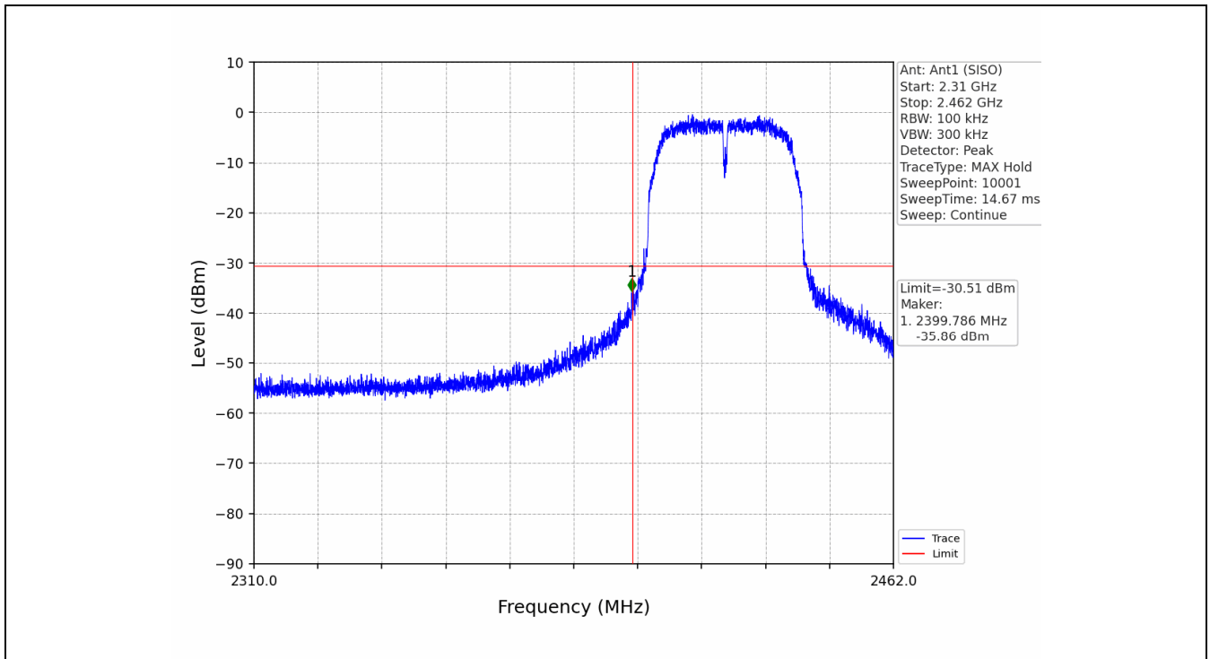
802.11n(HT40)_LCH_2422MHz_Ant1 (SISO)_NTNV
