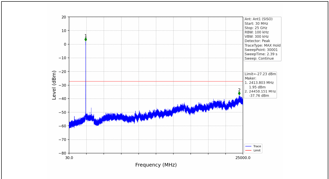
802.11n(HT20)_MCH_2437MHz_Ant1 (SISO)_NTNV
