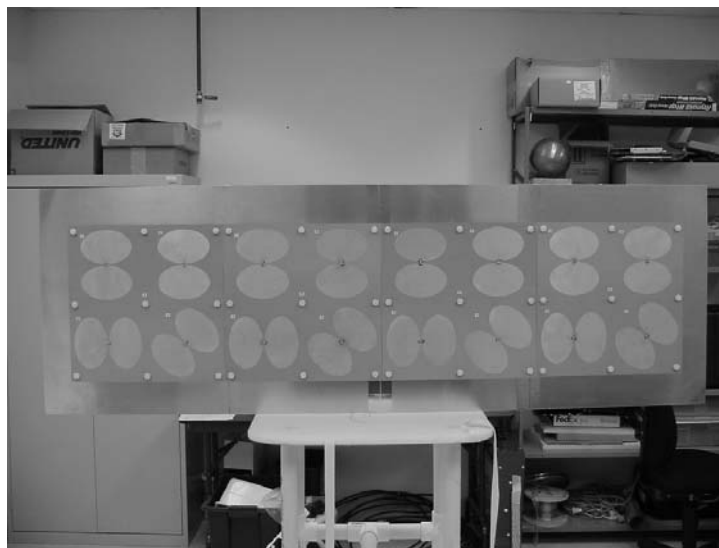
Antenna array
