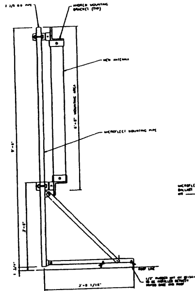
SECTION I N.E.S.
