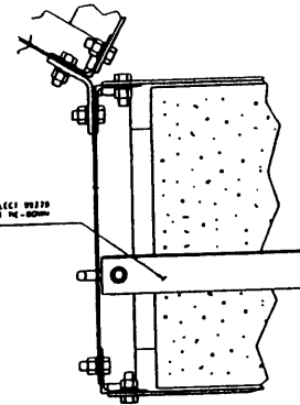
DETAIL "A" N.E.S.
