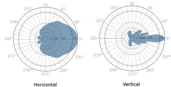
ZDADJ700-14-60Patterns
