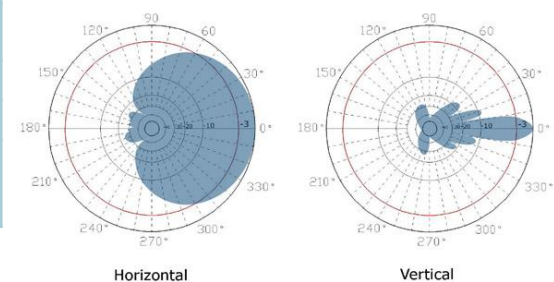
ZDADJ700-12-120 Patterns
