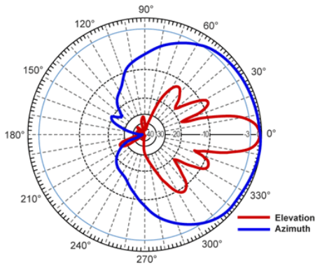
-45° - 2400 MHz
