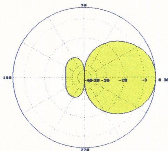
SAM-237R E-Plane
