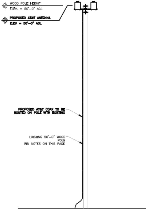
1 PROPOSED SITE 1 ELEVATION SCALE: N.T.S.
