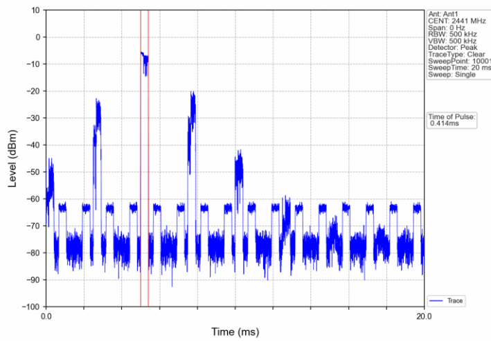
8DPSK_3DH1_HOPP_Ant1_NTNV
