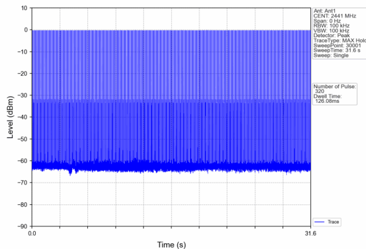
GFSK_DH1_HOPP_Ant1_NTNV
