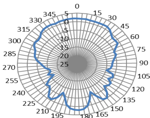
XZ-2450MHz
