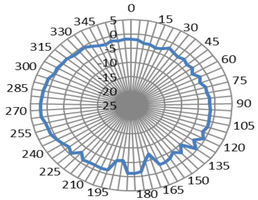
YZ-5500MHz
