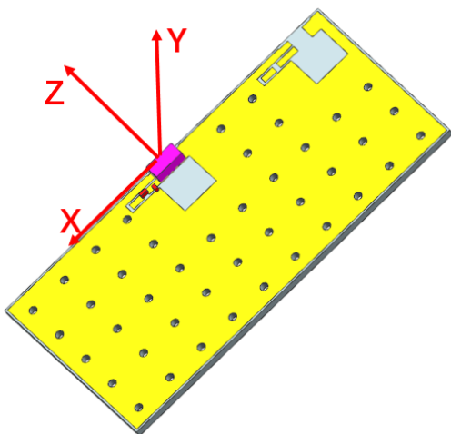
XZ-2450MHz
