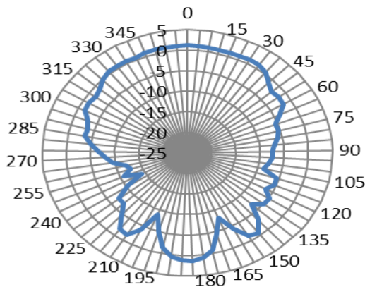
XZ-2450MHz
