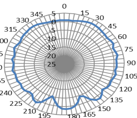
YZ-2450MHz
