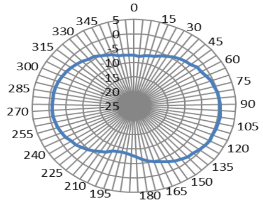
XY-2450MHz
