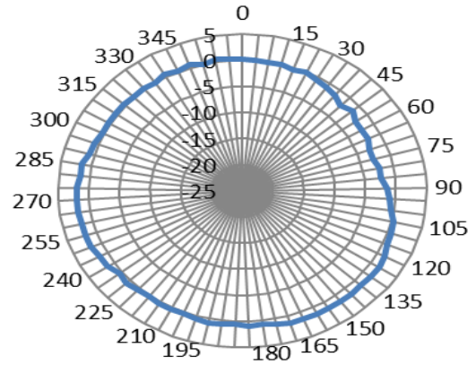
XY-5500MHz
