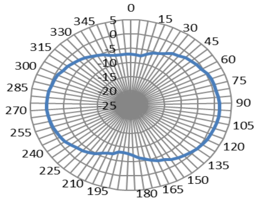
XY-2450MHz
