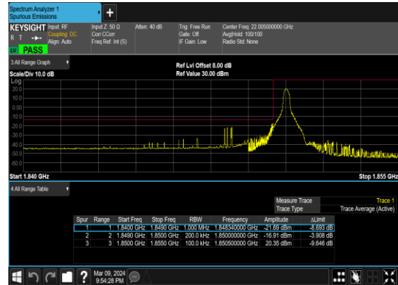
N2(20M)_DFT-s-OFDM_BPSK_Edge_1RB_Left_Low_CH
