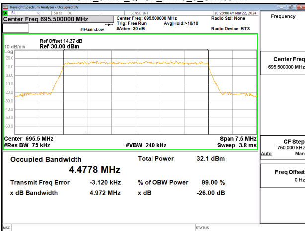
Band71_5MHz_QPSK_RB25_0_CH133447
