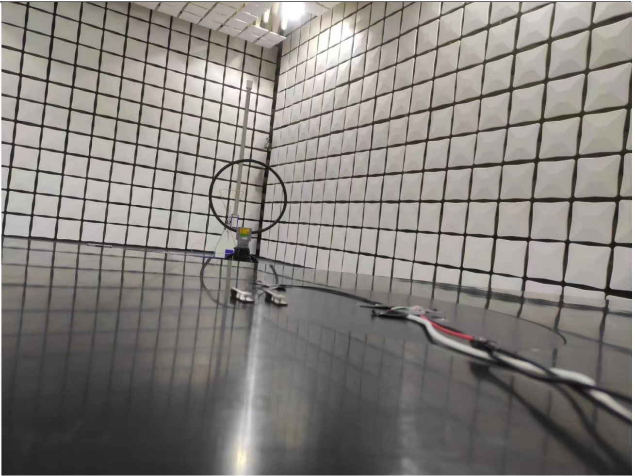
RE9KHz~30MHz
