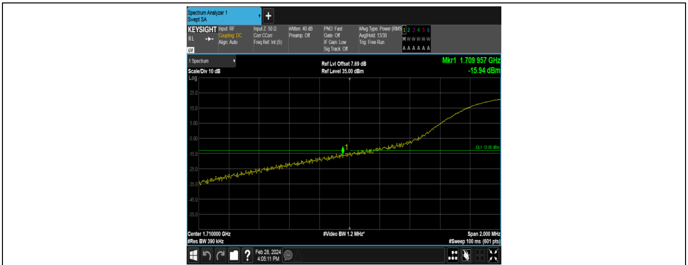
Band4-20MHz-QPSK-20050-1RB#99
