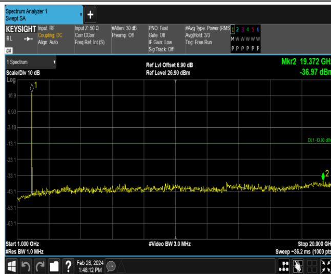
Band2-5MHz-QPSK-18900-1RB#0-Range2:1000~20000MHz
