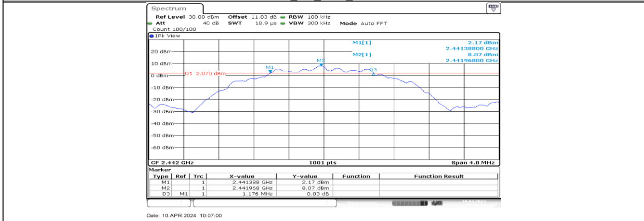
BLE_2M_Ant1_2442
