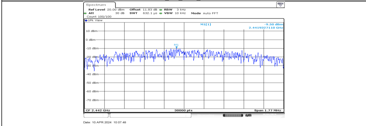
BLE_2M_Ant1_2442
