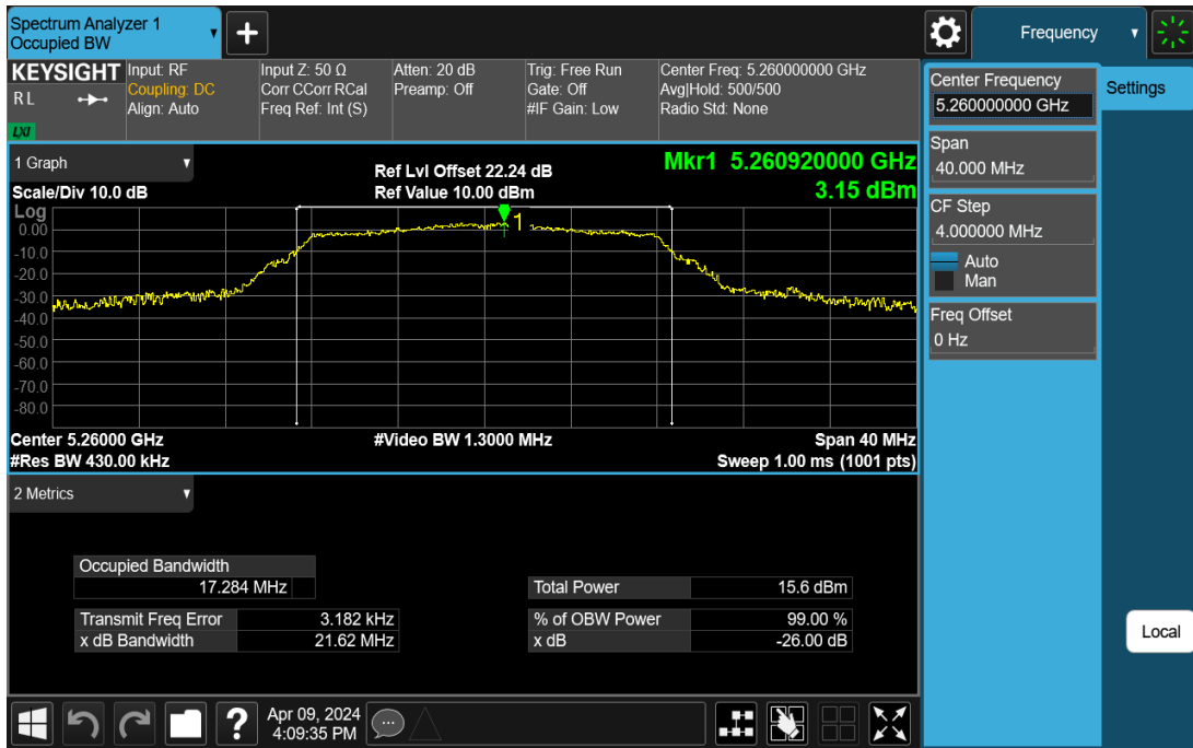
11A-Ant1-5260
