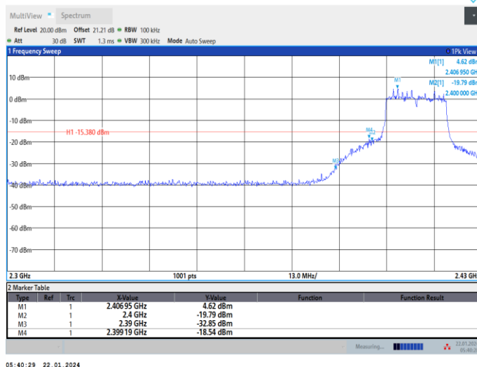
11G_Ant1_Low_2412
