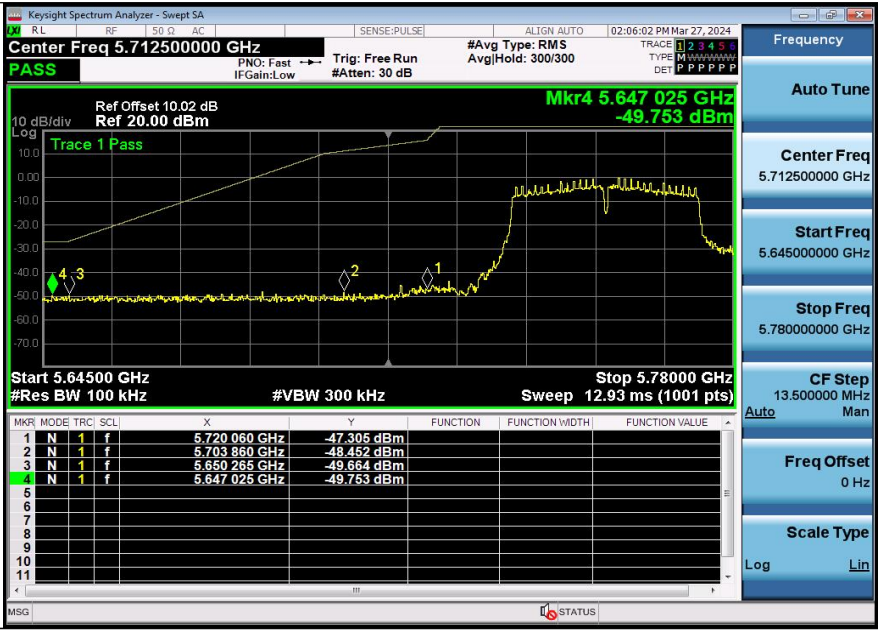
11N40ISO-Ant3-5755-PASS
