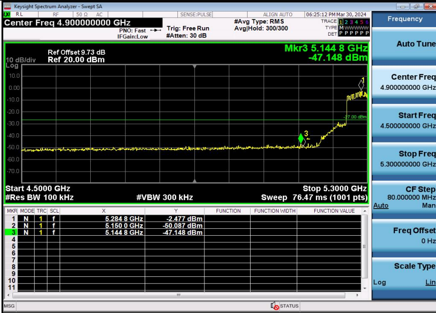
11AX80SISO-Ant3-5290-PASS
