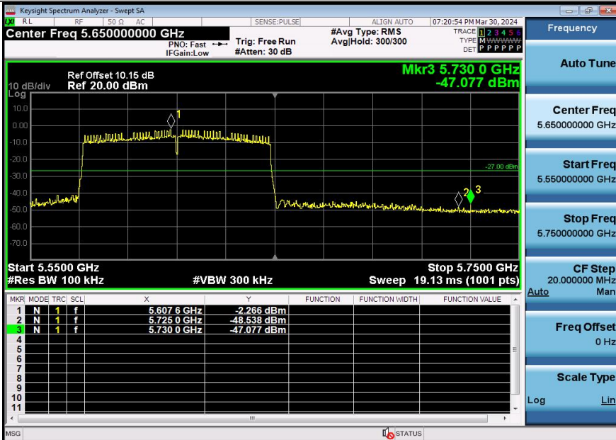
11AX80SISO-Ant3-5610-PASS
