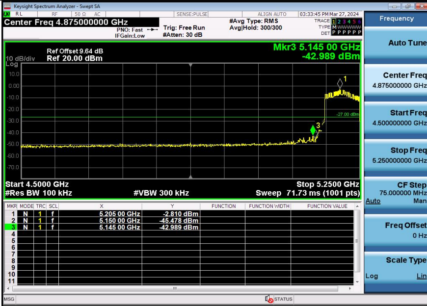
11AX80SISO-Ant3-5210-PASS
