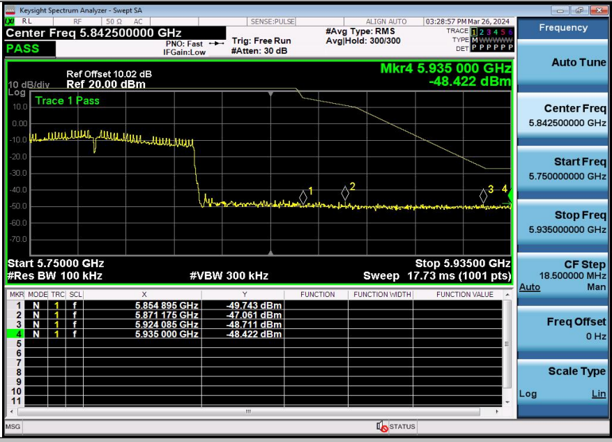
11AX80SISO-Ant1-5775-PASS
