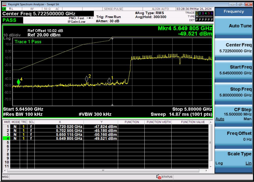
11AX80SISO-Ant1-5775-PASS
