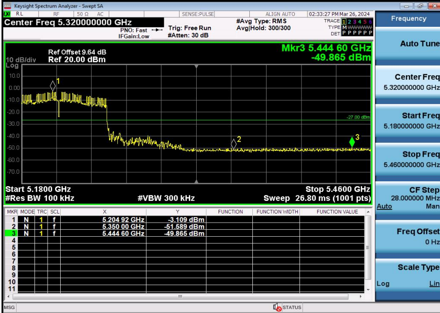
11AC80SISO-Ant1-5210-PASS
