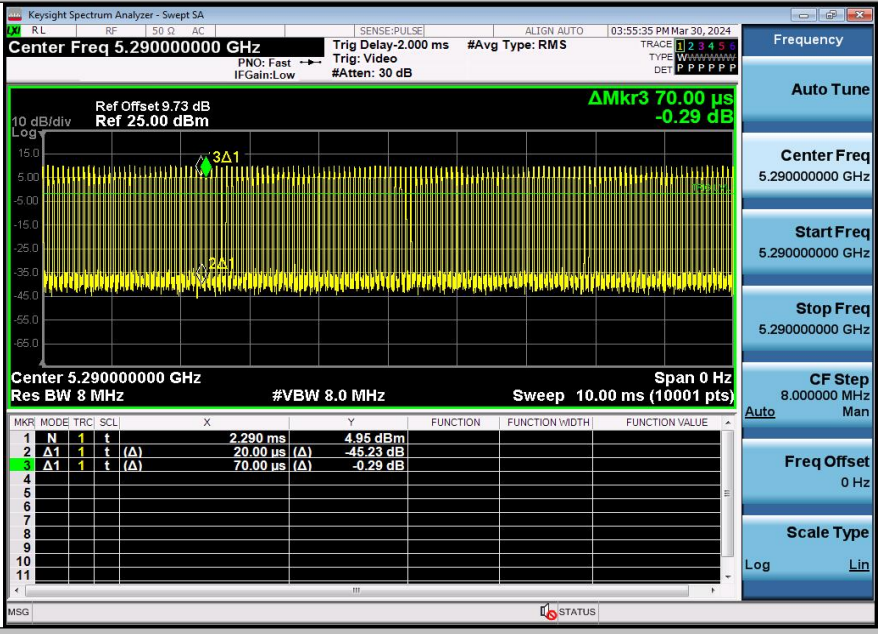
NTNV-11AC80SISO-Ant2-5290
