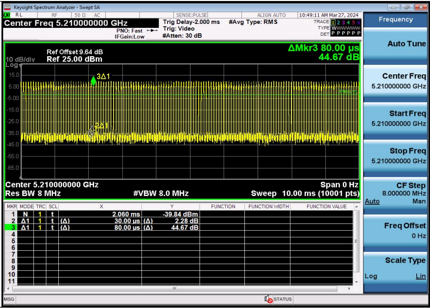
NTNV-11AC80SISO-Ant2-5210
