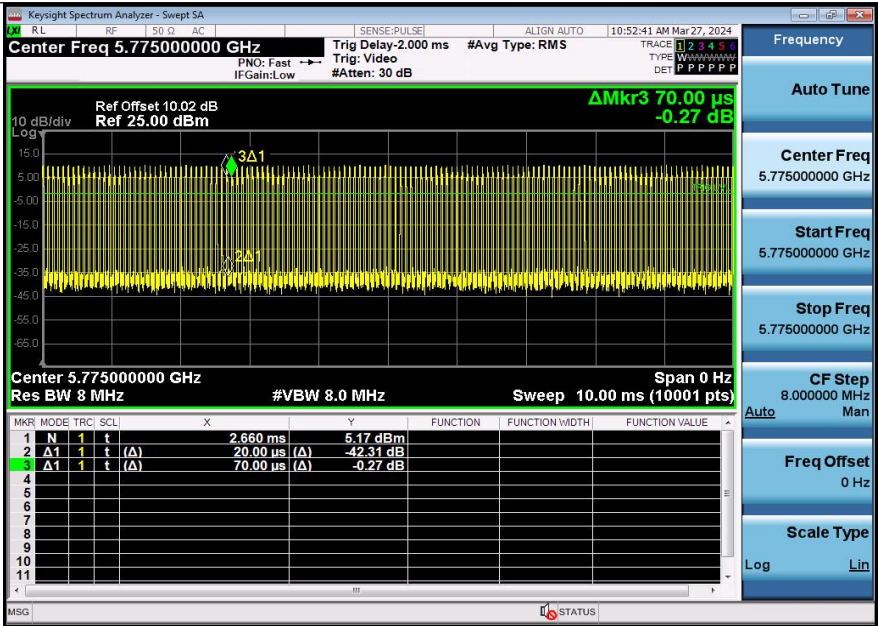
NTNV-11AC80SISO-Ant2-5775
