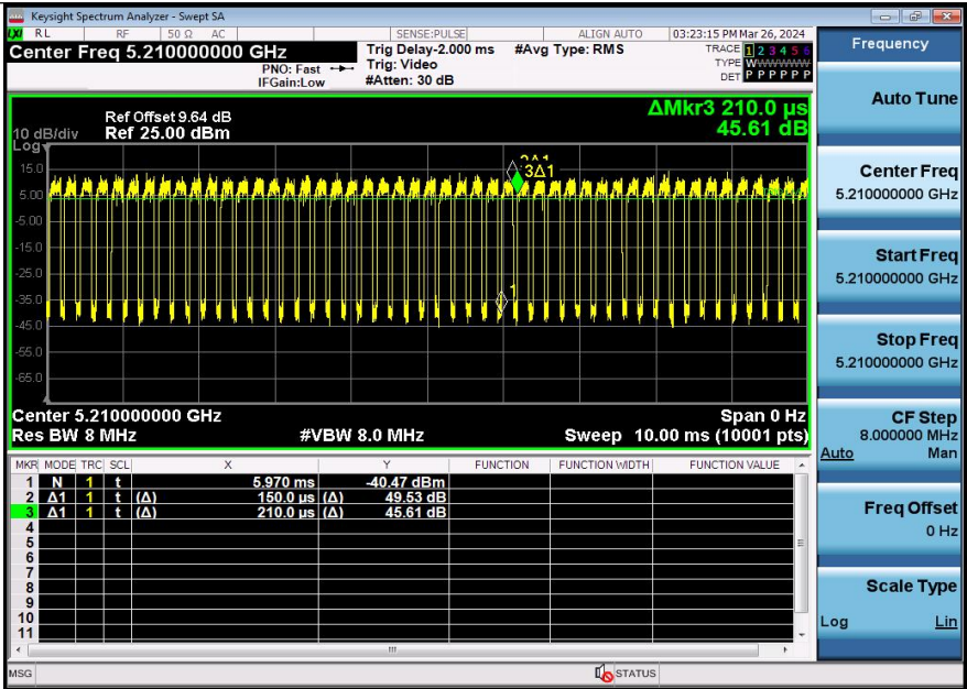
NTNV-11AX80SISO-Ant1-5210
