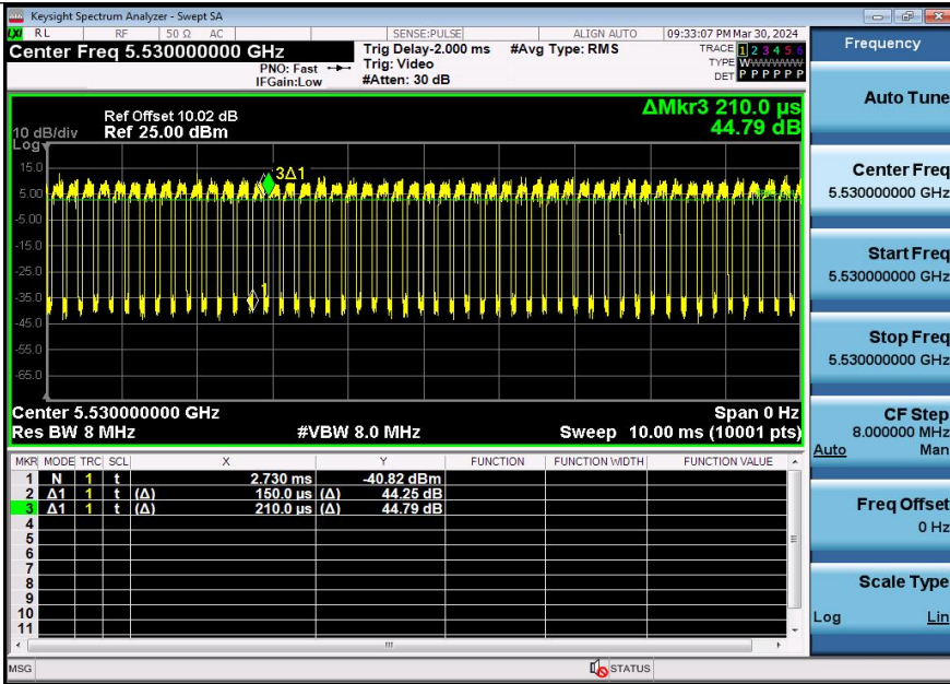
NTNV-11AX80SISO-Ant1-5530
