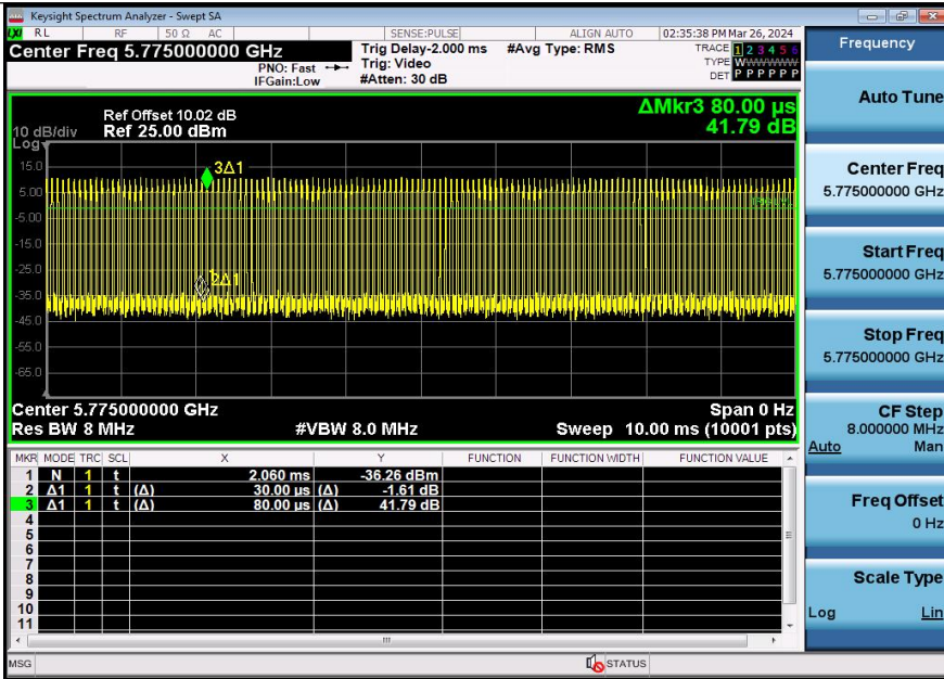
NTNV-11AC80SISO-Ant1-5775
