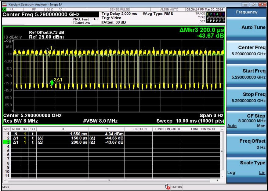
NTNV-11AX80SISO-Ant1-5290
