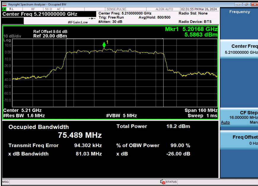
11AC80SISO-Ant1-5210
