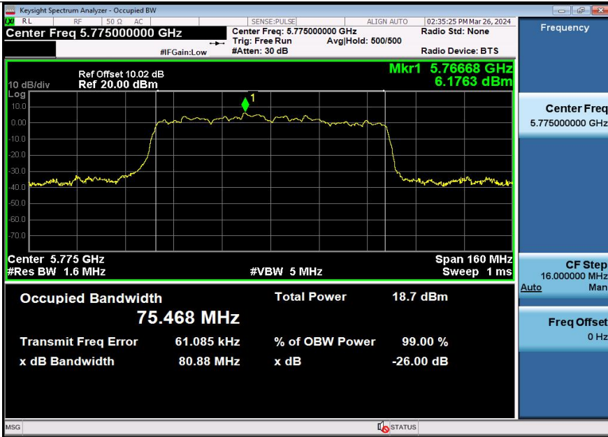
11AC80SISO-Ant1-5775
